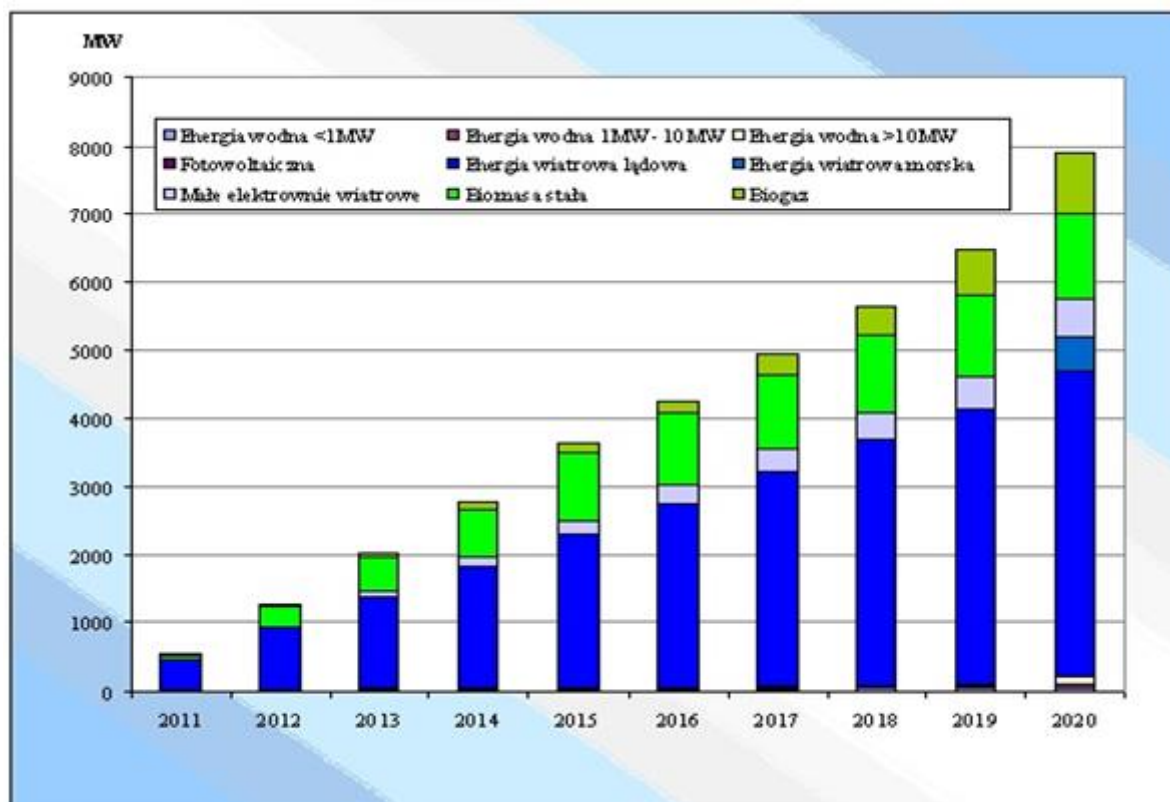
Rysunek 35 Prognozowany przyrost mocy elektrycznych zainstalowanych w OZE w latach 2011-2020 w [MW],
